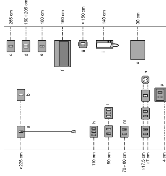
Fig. 14 – Quote installative di prese a spina e apparecchi di comando (in cm e riferite alla mezzaria del dispositivo). a - prese a spina e comandi per doccia e vasche da bagno; b - pulsanti per alimentazione ventole di aspirazione bagno; c - presa a spina per alimentazione cappa cucina; d - suoneria; e - passacavo per alimentazione scaldia acqua; f - quadri unità abitative; g - prese a spina e comandi in autorimesse e cantine; h - prese a spina e comandi per interno bagni e piano di lavoro cucina; i - citofoni; l - comandi di punti luce, prese a spina ecc.; m - prese a spina e comandi punti luce a testaleto; n - prese a spina, prese per TV - radio, telefono ecc.; o - prese a spina per prese a parete (incassate o sporgenti); p - prese a spina su canalina battiscopa; 7 cm per prese a spina su canalina battiscopa; 17,5 cm per prese a parete (incassate o sporgenti); 7 cm per prese a spina su canalina battiscopa; o - cassette di derivazione; p - prese a spina installate su torrette sporgenti dal pavimento.
